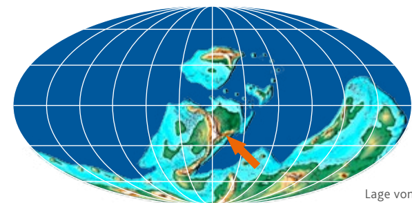
Lage von Rheinland-Pfalz im Devon, (1)
