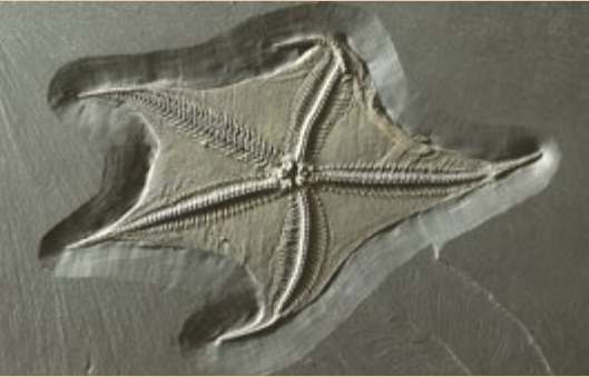
Schlangensterne ( Loriolaster mirabilis ), Bundenbach, (4)
