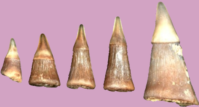
Raubfischzähne ( Saurichthys sp. ), Palzem
