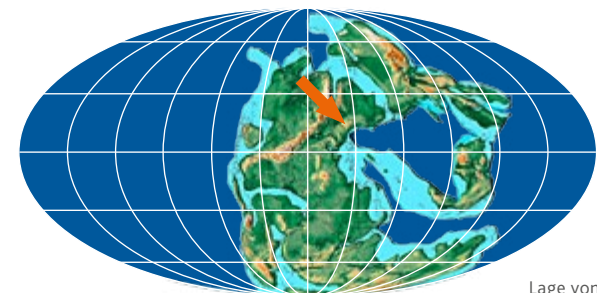
Lage von Rheinland-Pfalz im Perm, (1)
